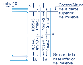
Dimensiones del espacio recomendadas para instalación de puerta fija
